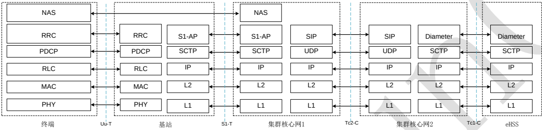
图5 控制面协议栈
