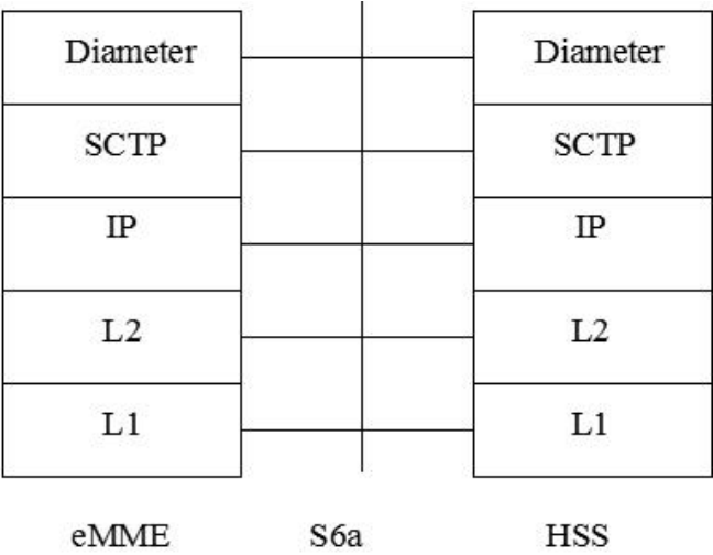
图17 S6a 接口协议栈
