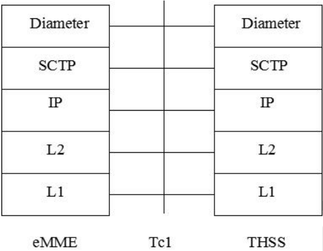
图19 Tc1 接口的协议栈
