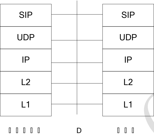
图11 D 接口控制面协议栈
