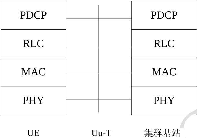
图9 Uu-T 接口用户面协议栈
