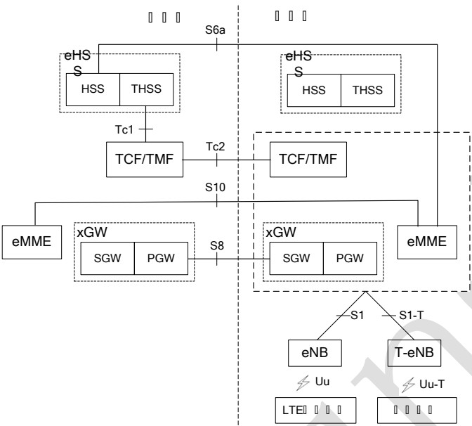
图4 漫游架构
