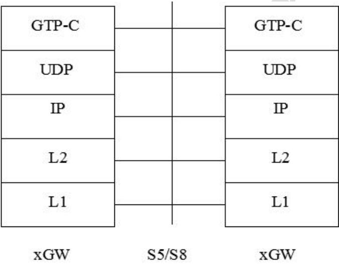
图16 S5/S8 接口控制面协议栈
