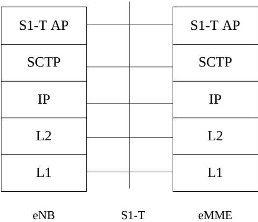
图13 S1-T 接口控制面协议栈
