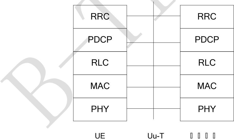
图8 Uu-T 接口控制面协议栈
