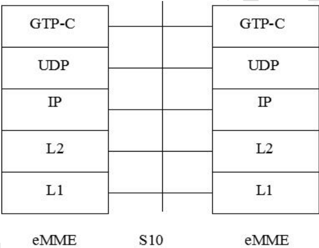
图18 S10 接口协议栈
