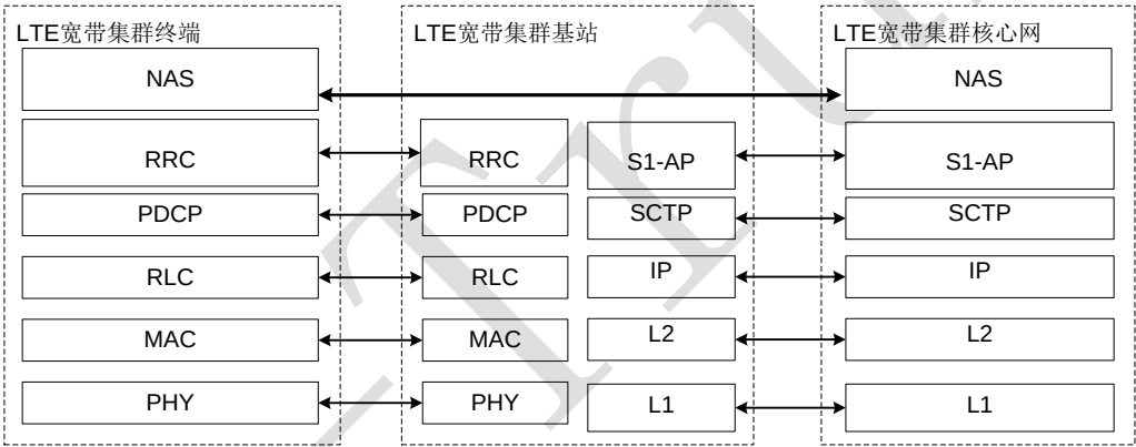
图10 集群 NAS 接口协议栈
