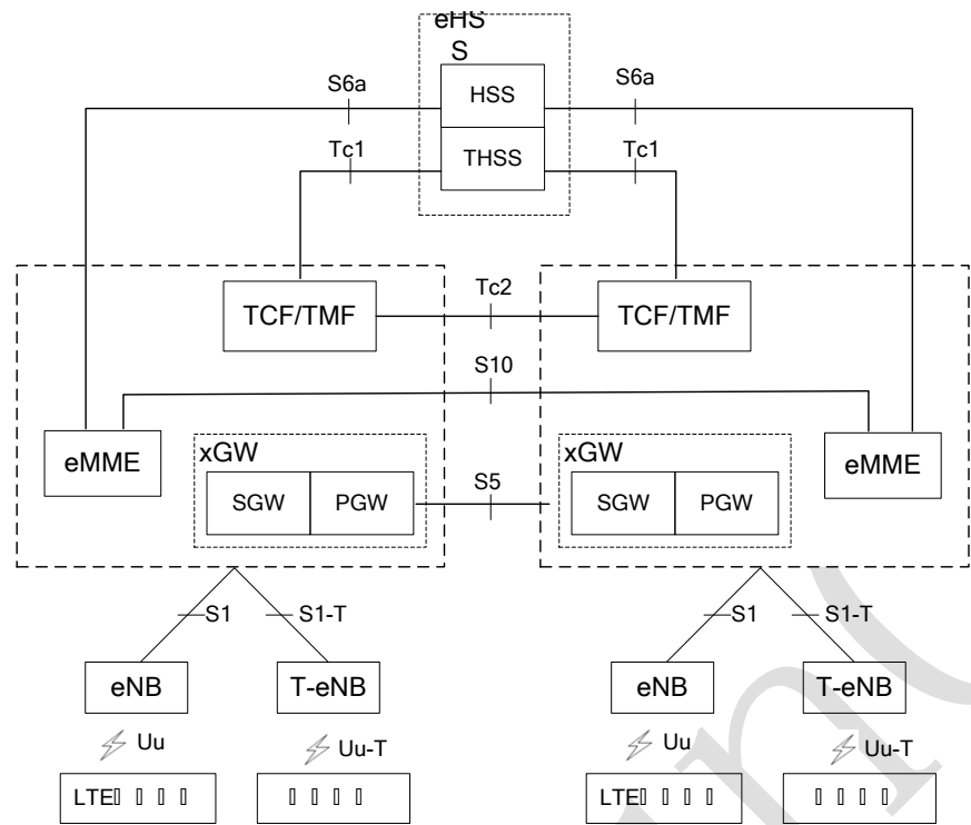
图2 本地网架构-多核心网
