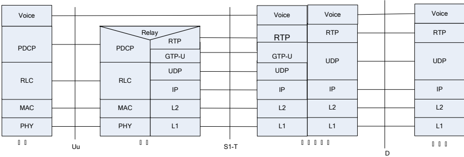
图7 AMR over PDCP 的用户面协议栈（可选）
