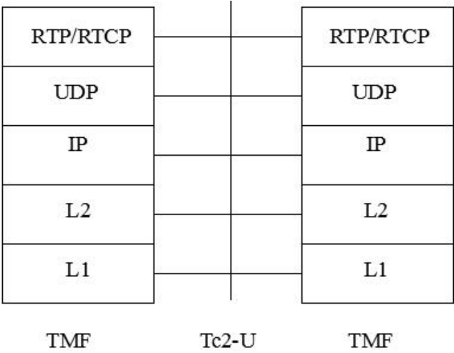
图21 Tc2 接口的用户面协议栈
