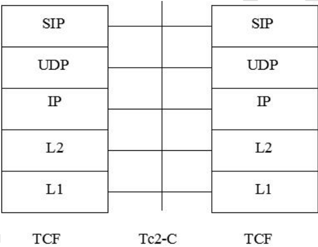
图20 Tc2 接口的控制面协议栈
