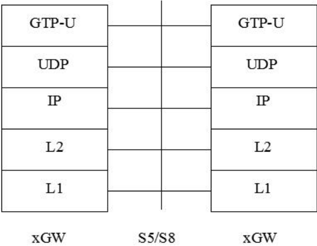
图15 S5/S8 接口用户面协议栈
