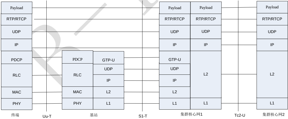
图6 用户面协议栈
